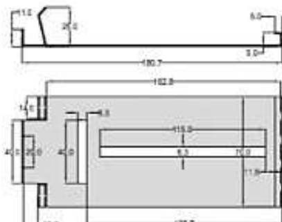
Clip pour bord vertical supérieur WEM8
